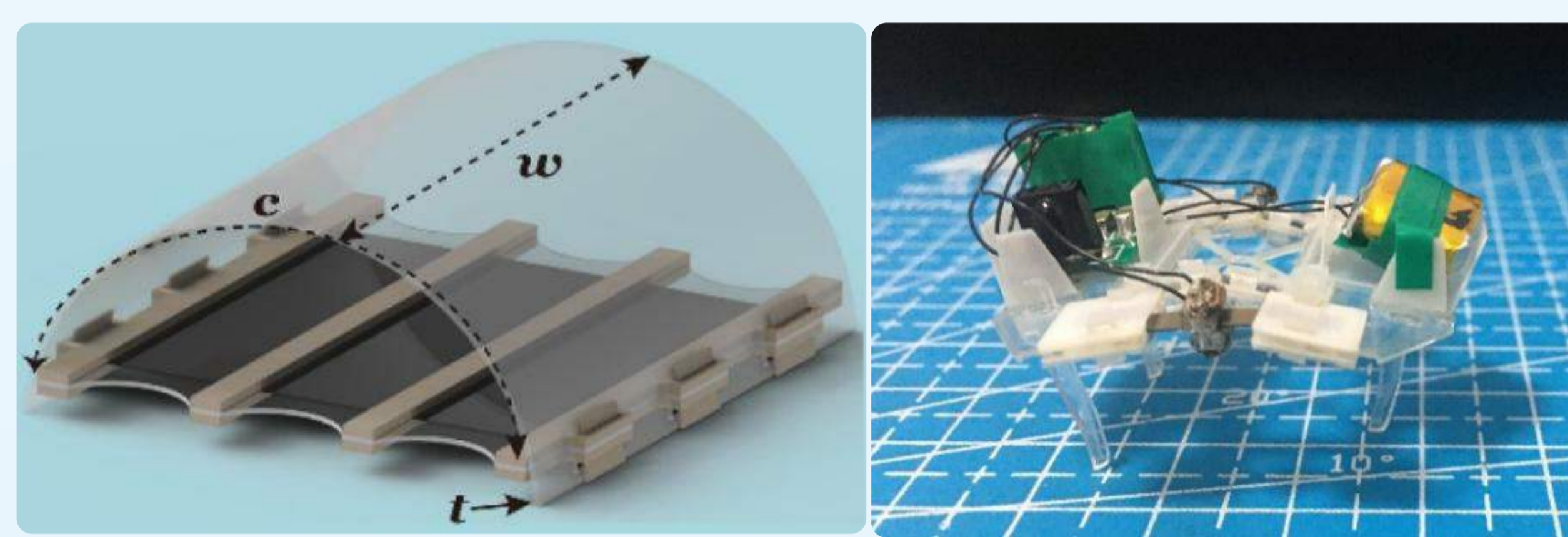
图1 微型刚柔软机器人
