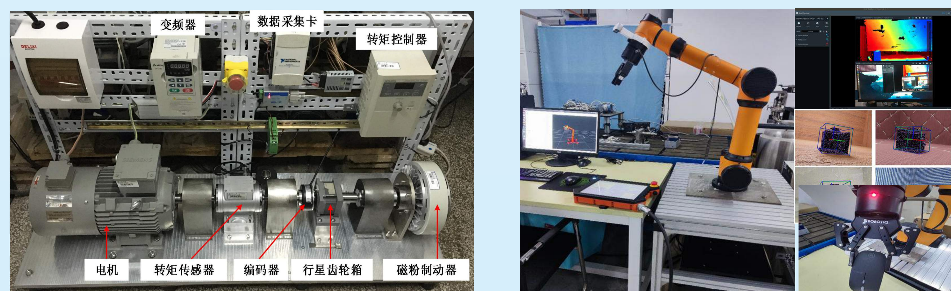
光纤光栅应变检测及其行星齿轮箱监测诊断
