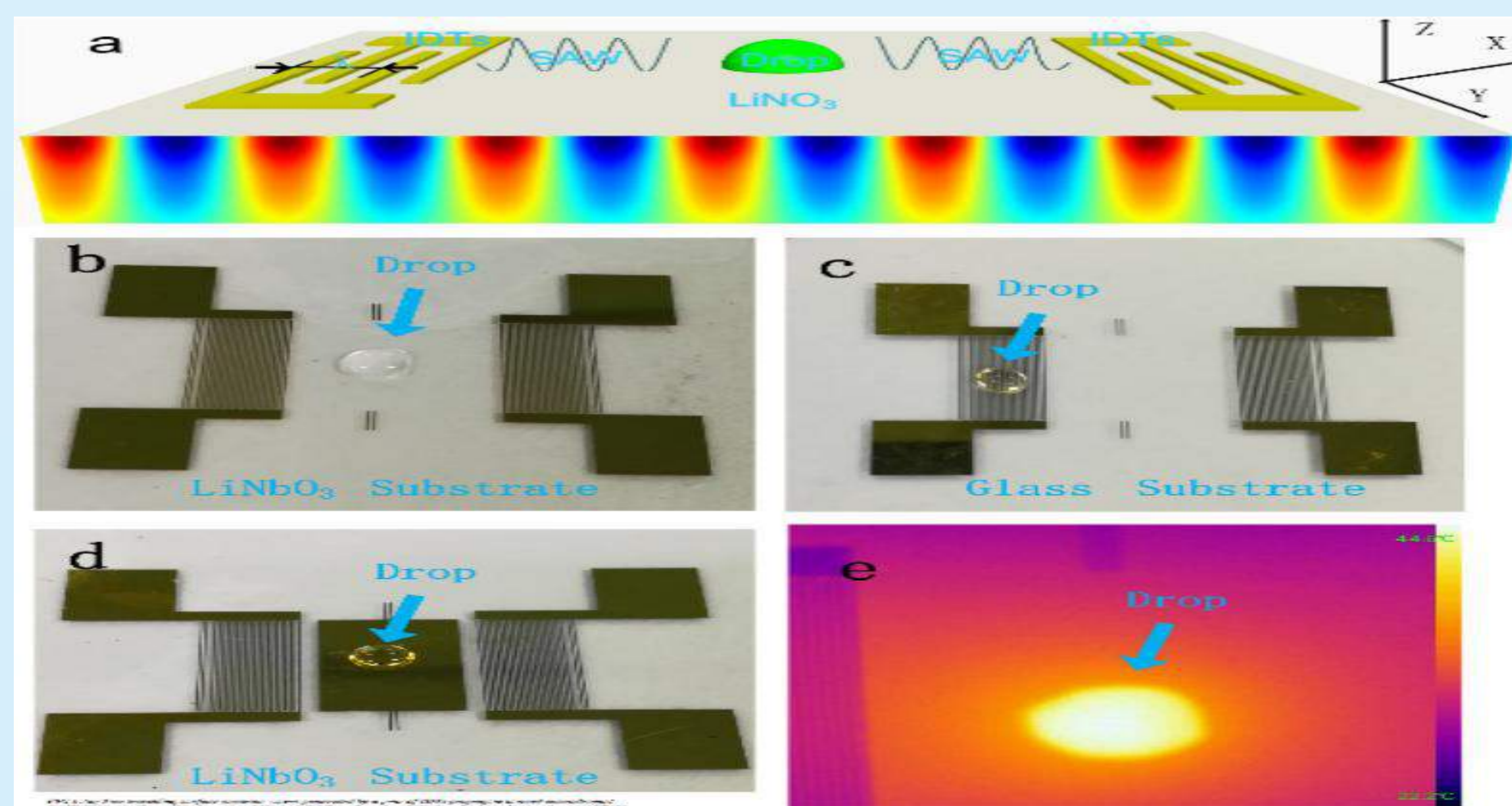
图5 微流控器件
